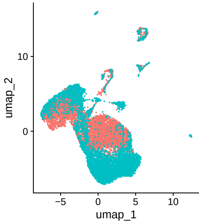
UMAP: restore
