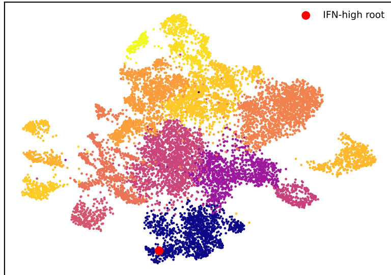
PAGA pseudotime
