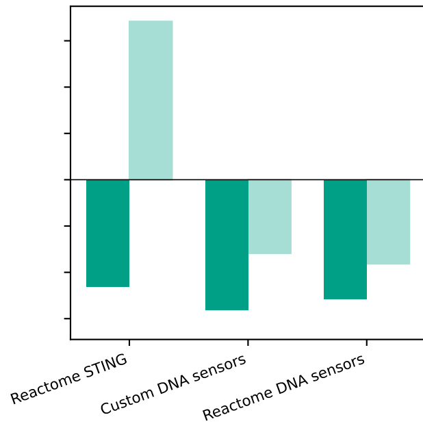
Ku80
