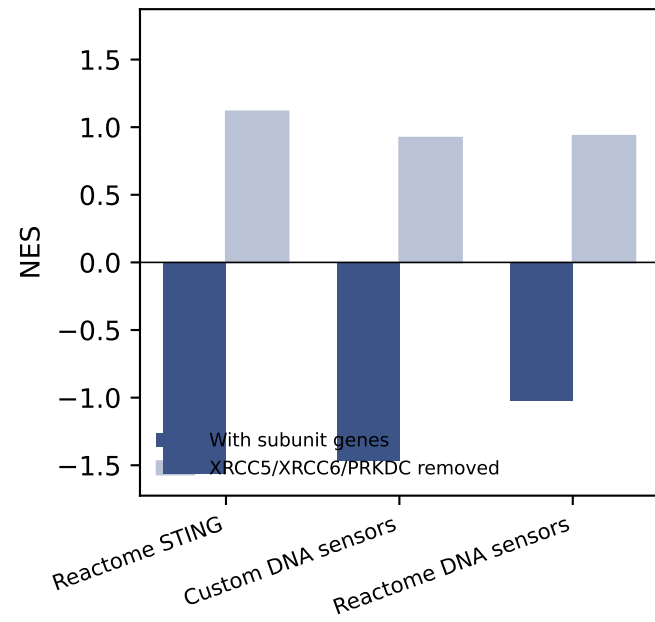
DNA-PKcs
