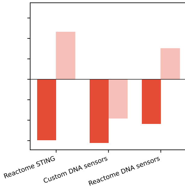
Ku70
