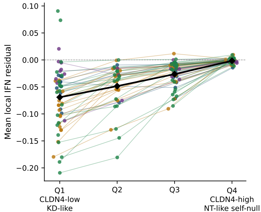
Hallmark IFN residual
