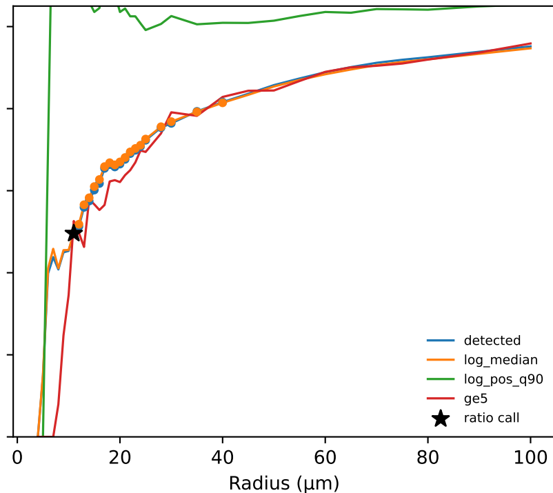
CD8+NK count
