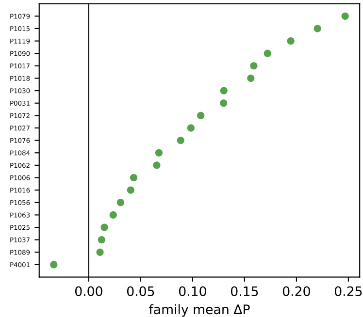
GSE205335
