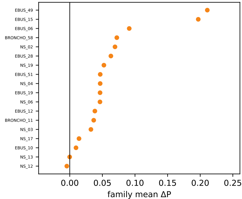
GSE131907
