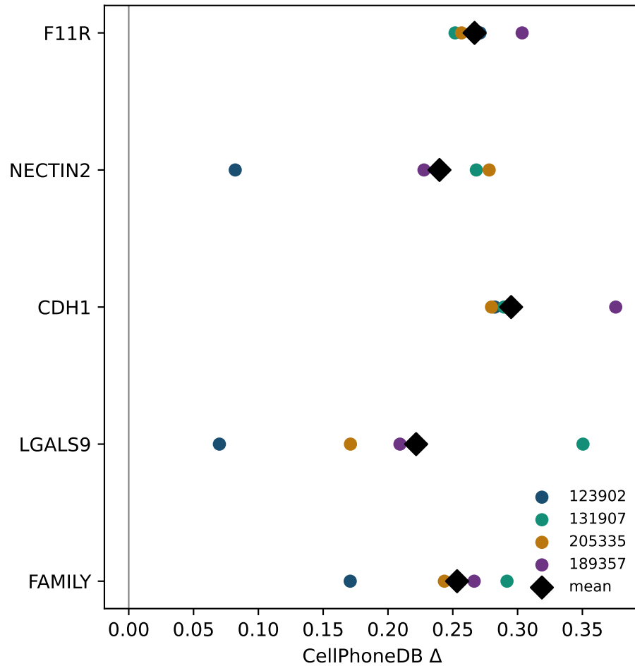
Winner pos_vs_neg expr_prop=0.10
