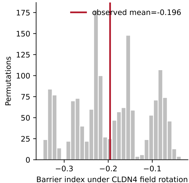
Rotate/shift null (CosMx)
