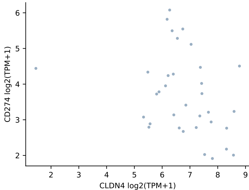
Lung (LUAD+LUSC) \rho=-0.354 p=0.0402 n=34
