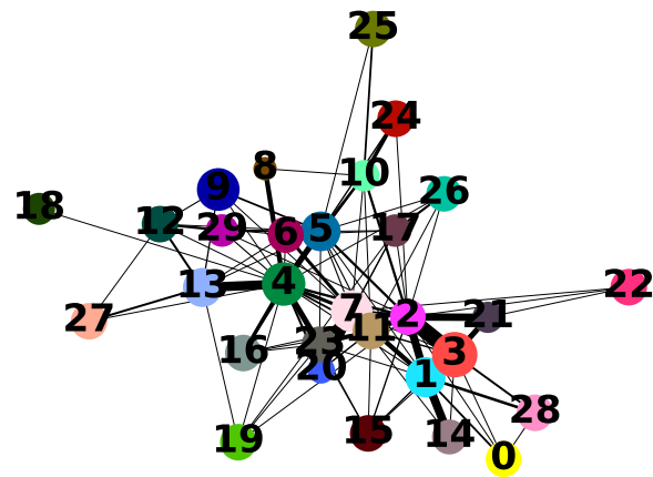
PAGA (Leiden)
