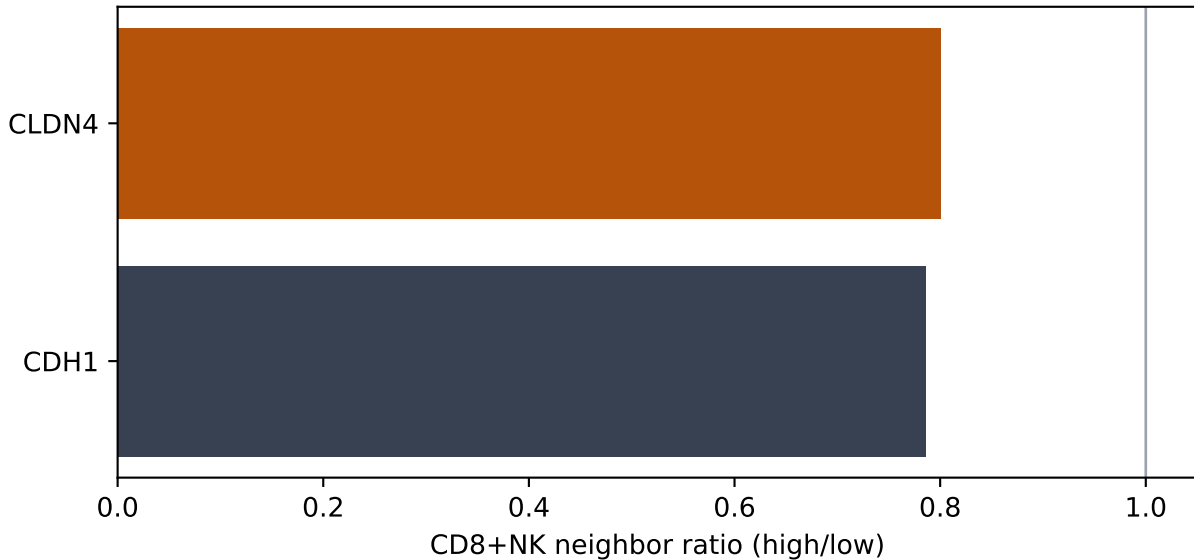
CosMx anchor_q4q1_50: q4_q1 @ 50 \mu m
