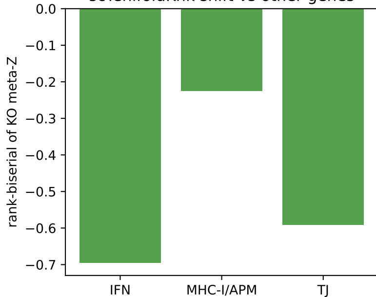
scTenifoldKnk shift vs other genes
