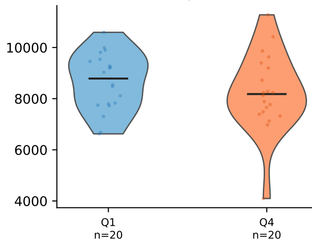
GSE31210 \delta=-799 p=1.2e-06
