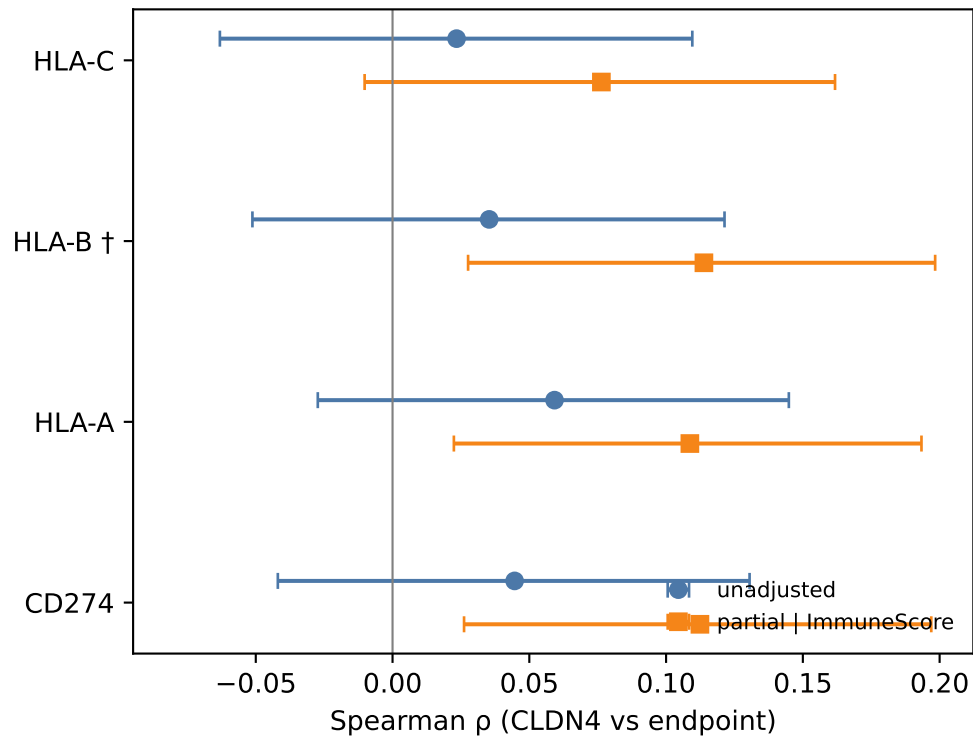
TCGA-LUAD n=515
