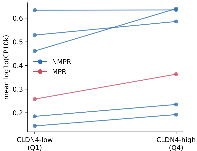
IFN (ISG core) module
