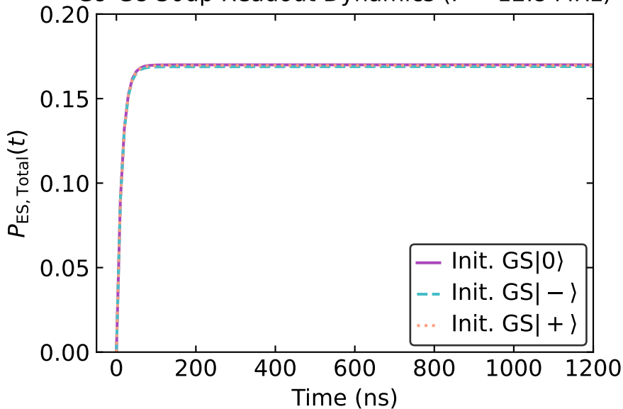
G9-G8 30dp Readout Dynamics ( \Gamma = 12.8 MHz)
