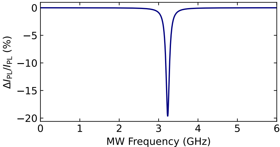
NV@Bulk ODMR Spectrum
