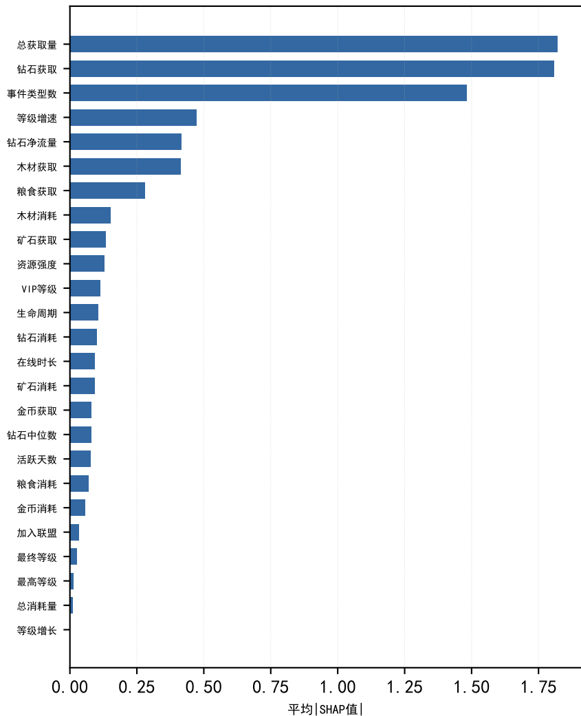
阶段1：付费概率驱动因子 (|SHAP|, 全部特征)
