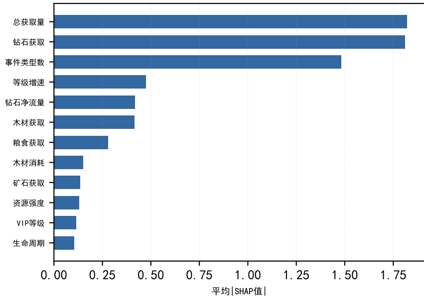
阶段1: 付费概率驱动因子 ( |SHAP| )
