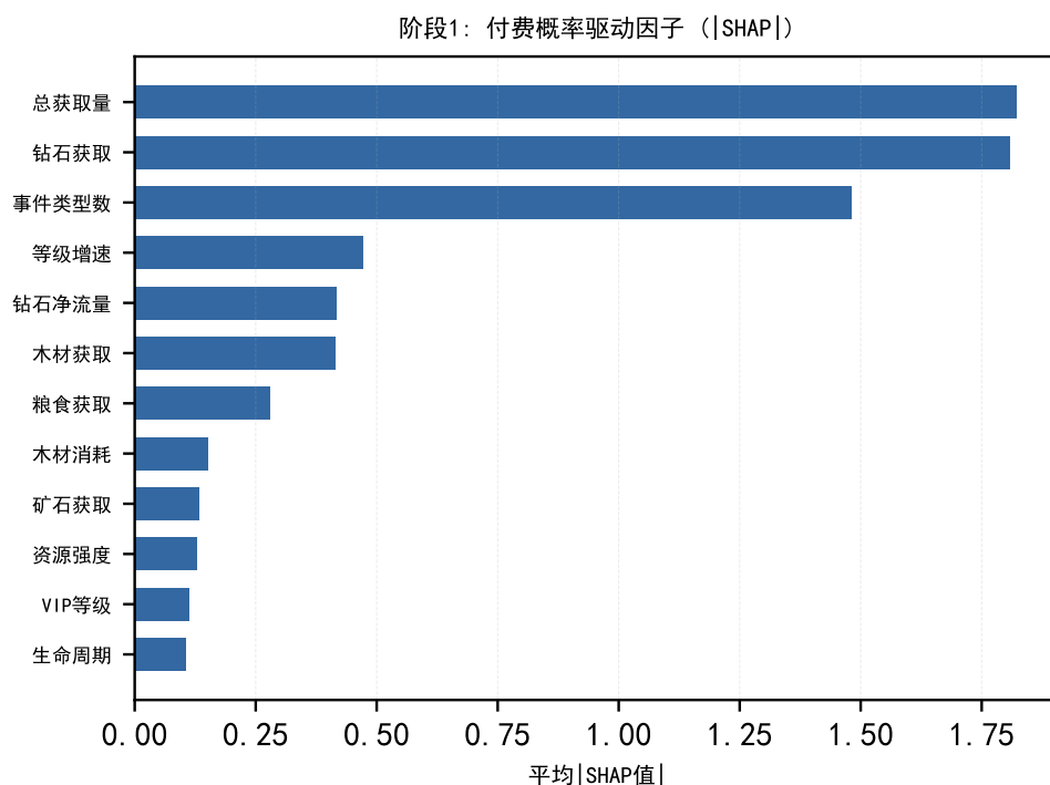
图 9: 阶段 1 XGBoost SHAP: 影响付费概率的关键因子
