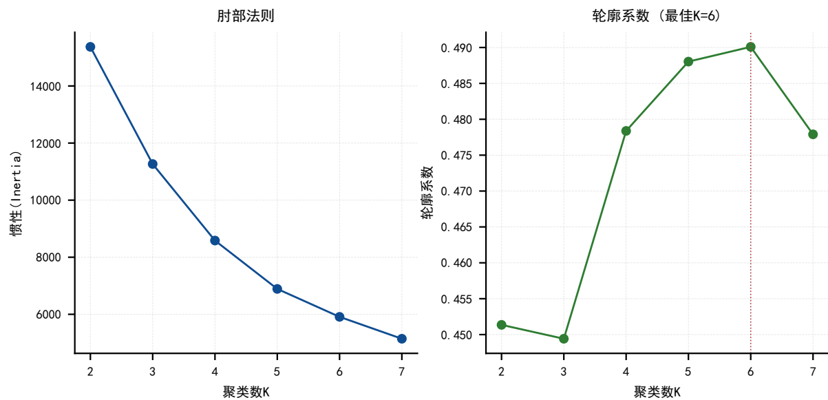
图 11: K-Means 肘部法则（左）与轮廓系数曲线（右，最佳 K = 6 ）
