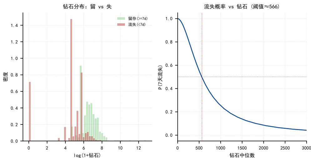
图 8: 钻石存量分布：留存 vs 流失玩家（左）与流失概率曲线（右）
