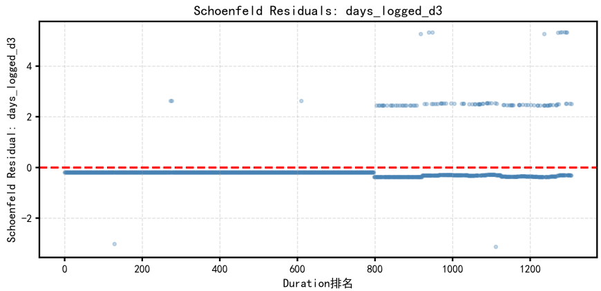
图 7: Schoenfeld 残差图: PH 假设违背最严重的协变量 (days_logged_d3)
