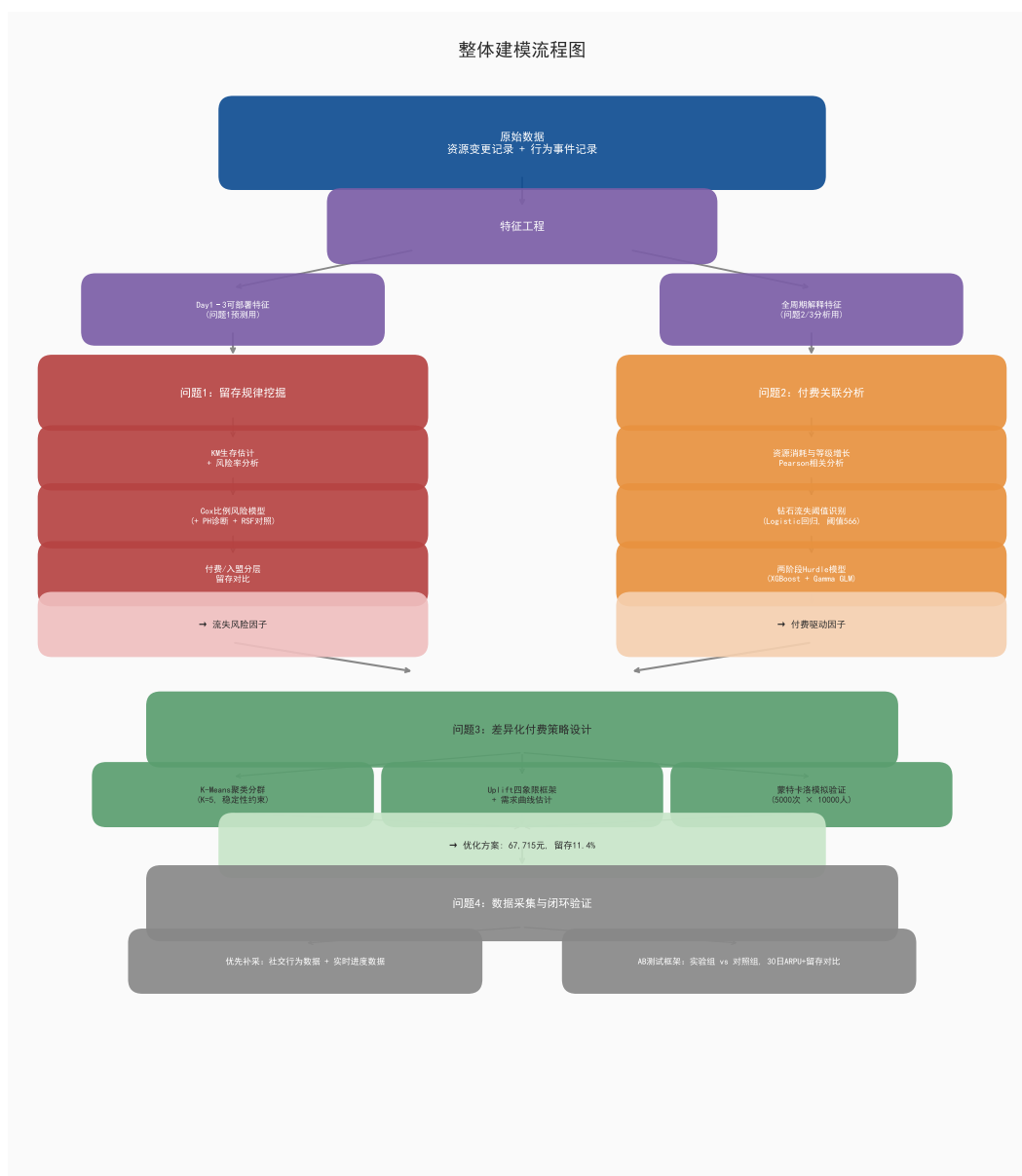
图 1: 整体建模流程图
