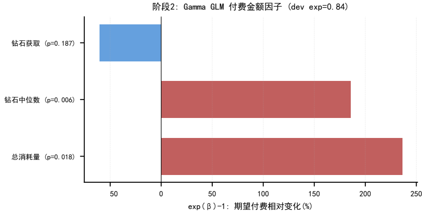
图 12: 阶段 2 Gamma GLM 系数：影响付费金额的关键因子 ( \exp(\beta) - 1 即期望付费相对变化%， p < 0.2 )
