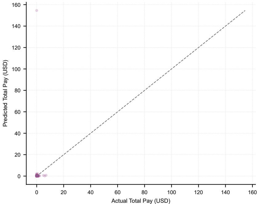
XGBoost: Predicted vs Actual (MAE=0.35 USD)
