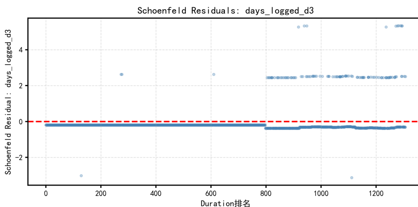
图 5: Schoenfeld 残差图: PH 假设违背最严重的协变量 ( \text{days\_logged\_d3} )
