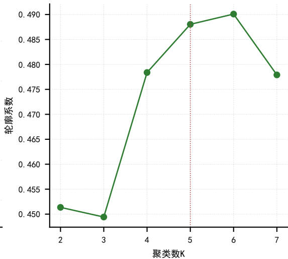
轮廓系数 (最佳K=5)
