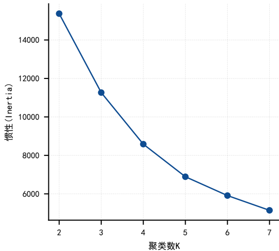
肘部法则
