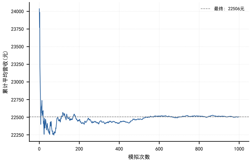
蒙特卡洛收敛曲线
