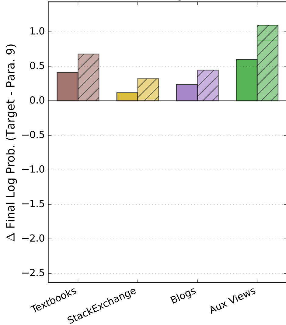
Data Strategies (7B)
