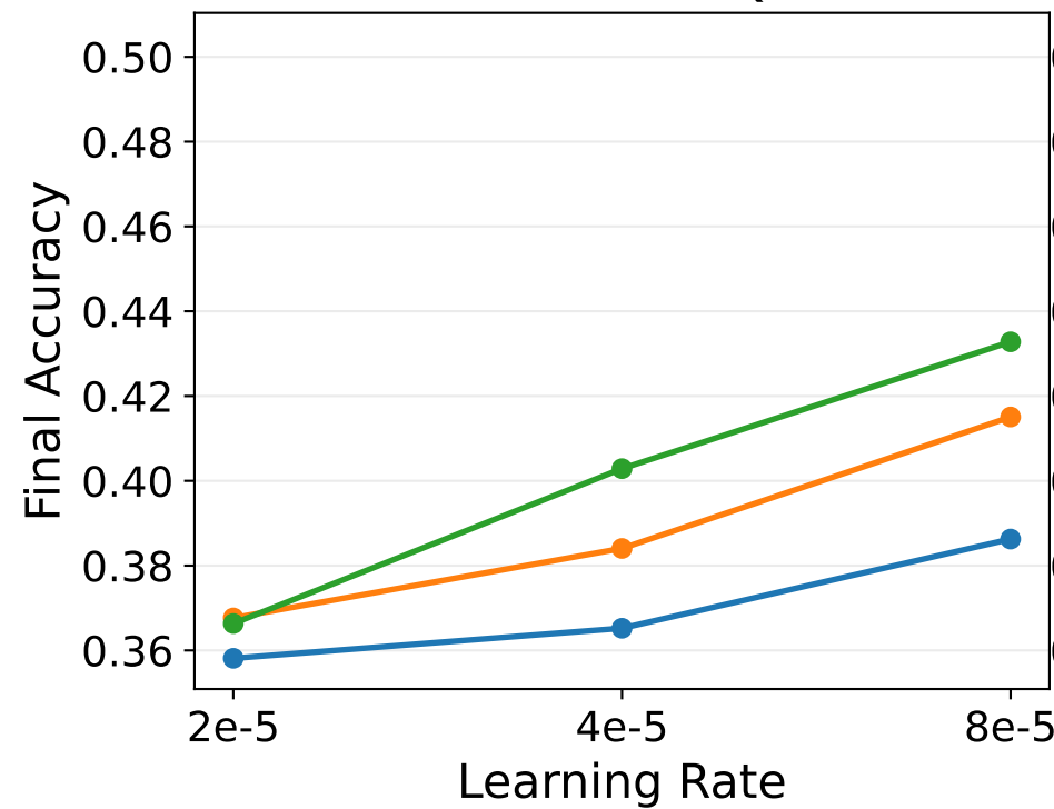
Factual MCQA
