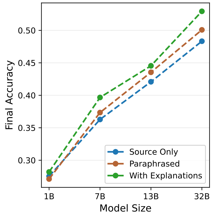
Factual MCQA
