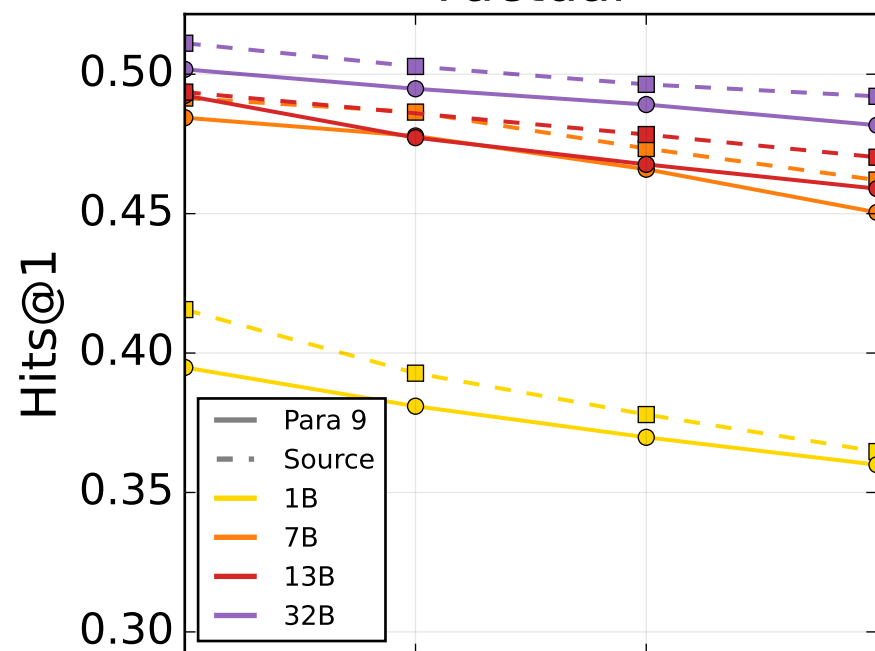
Factual
