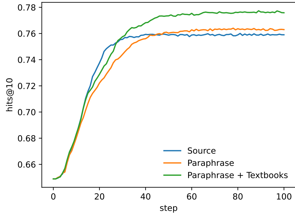
Factual Probes — hits@10
