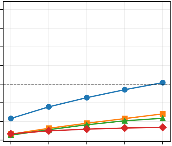
FromPlan
