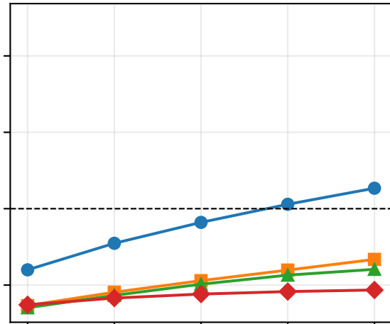
FromPlan
