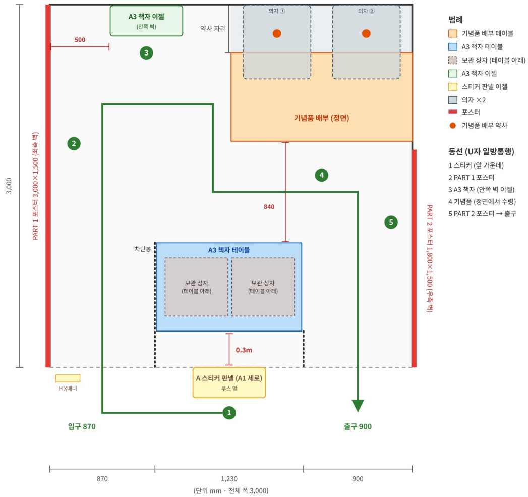
[그림 1] 부스 배치도 (단위 mm)
