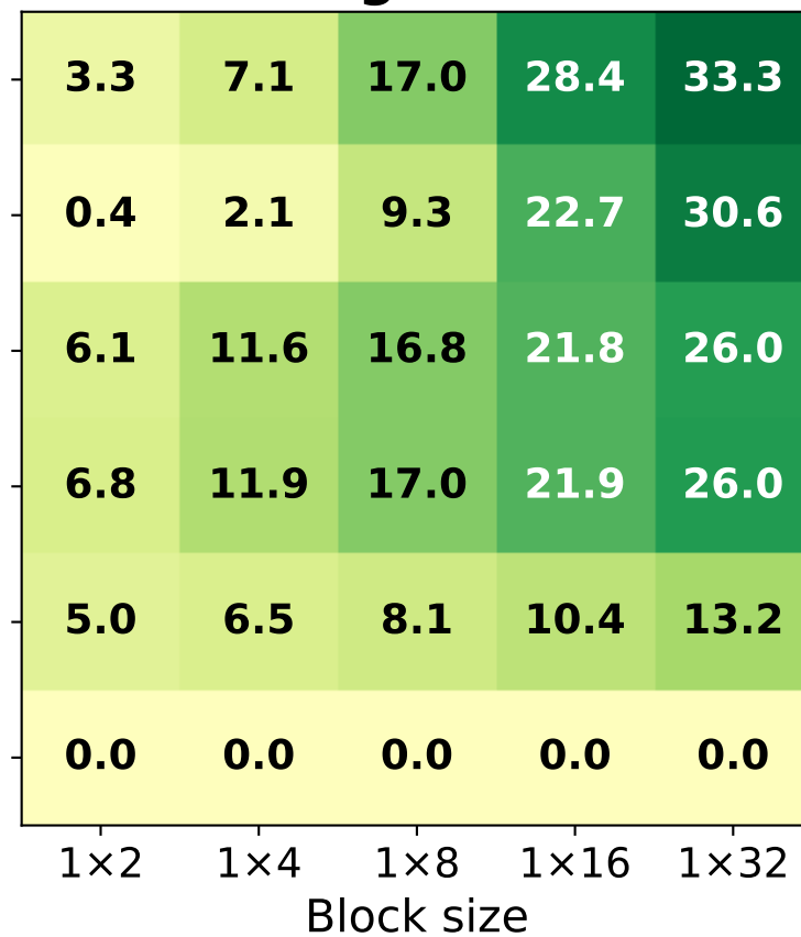
Larger ViT
