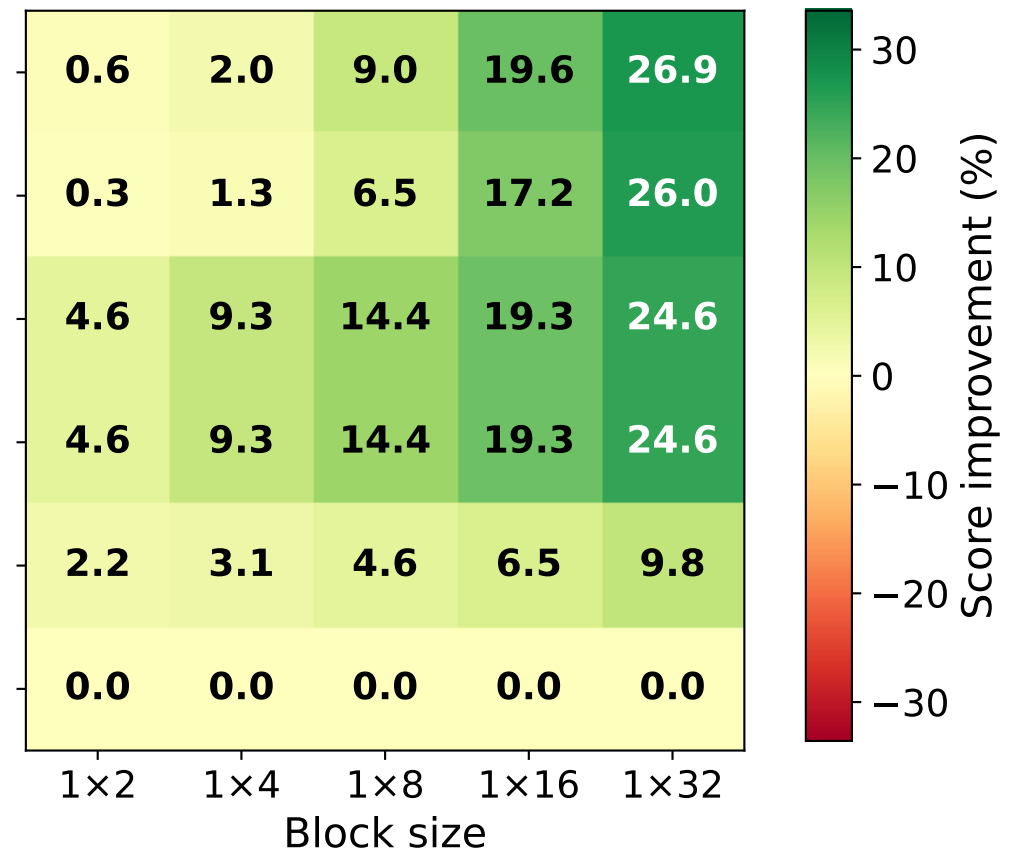
SmolLM2
