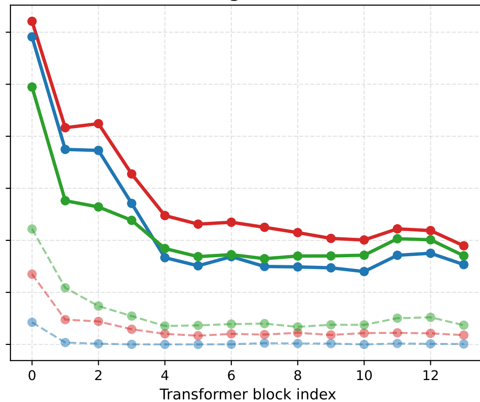
Larger ViT
