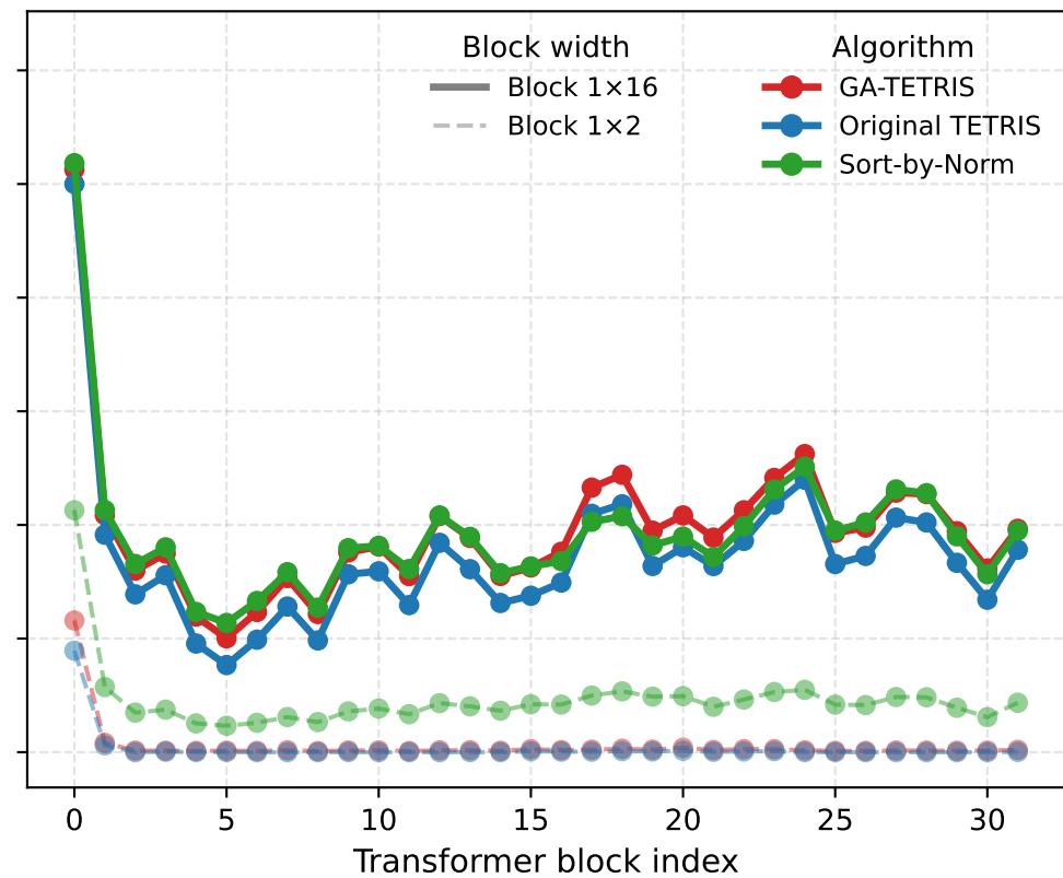
SmolLM2
