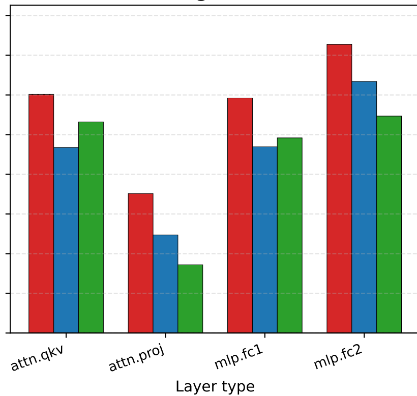
Larger ViT
