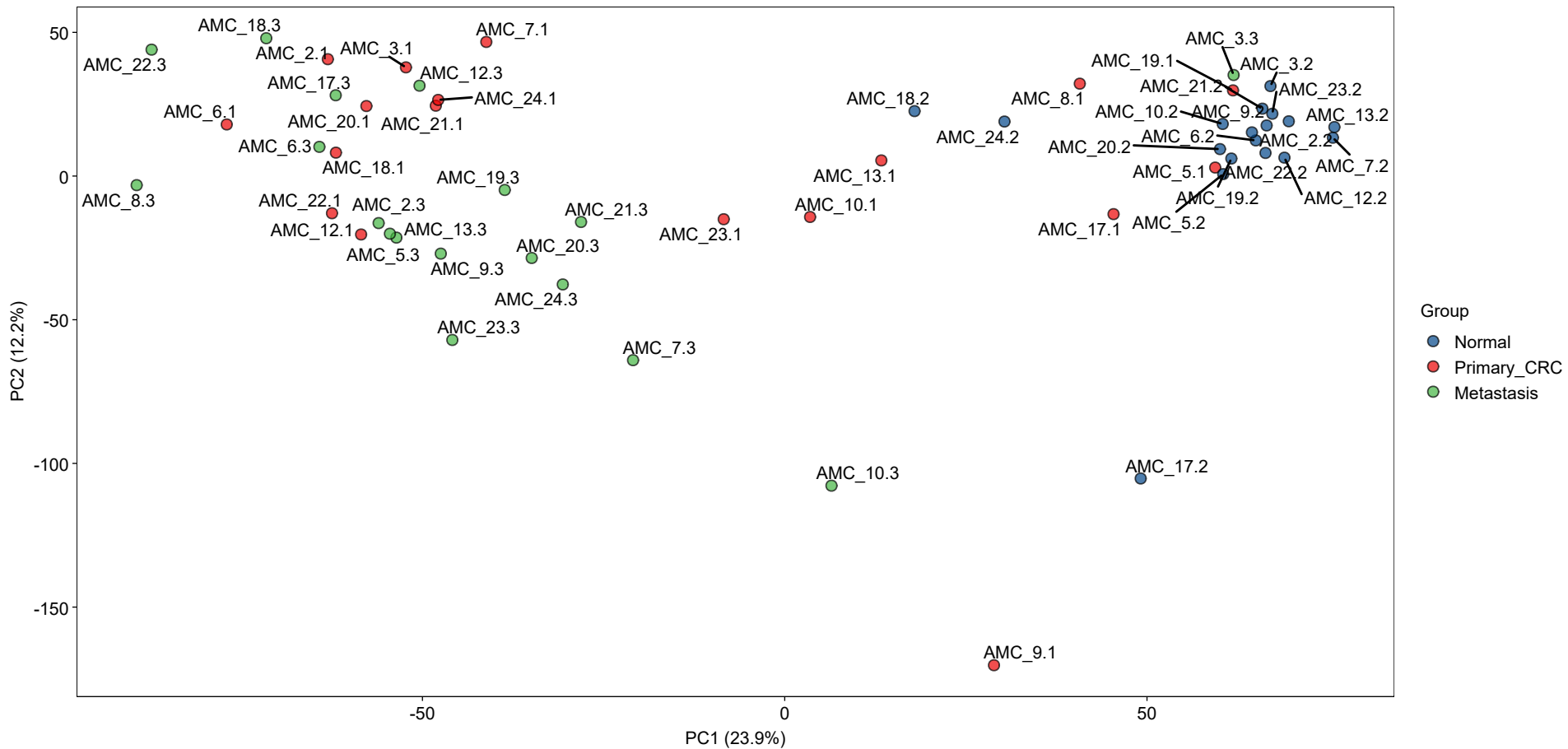
PCA of GSE50760
