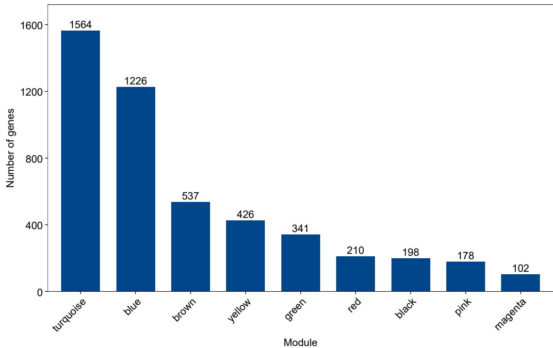
Module sizes
