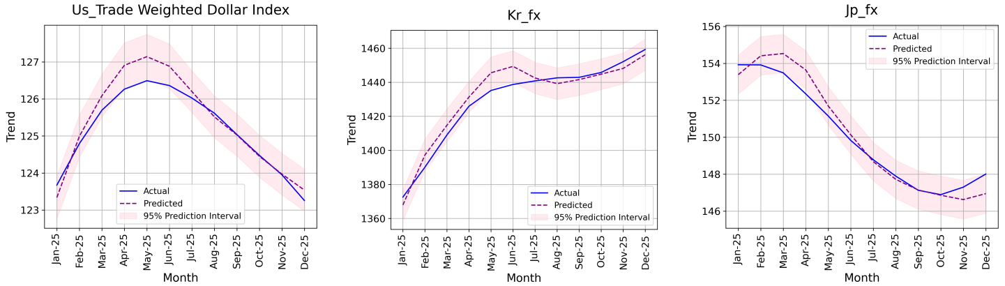
그림 2. B-MTGNN 평가 구간 성능 검증 (좌: 미국, 중: 한국, 우: 일본) Fig 2. B-MTGNN Performance Validation over the Evaluation Period (Left: US, Middle: KR, Right: JP)
