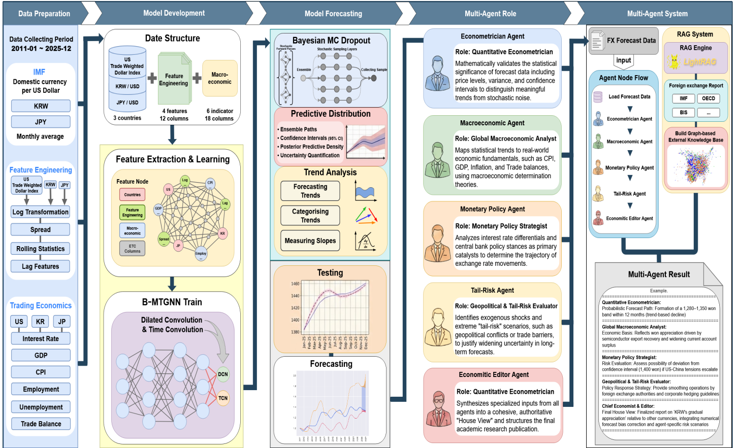
그림 1. 환율 예측 및 해석을 위한 AI 프레임워크. 본 파이프라인은 다변량 금융 및 거시경제 데이터 수집, 그래프 신경망 기반 베이저안 예측, 추세 및 환율 격차 분석, 그리고 멀티에이전트 해석을 통합하여 검증 가능하고 경제적 맥락에 기반한 의사결정을 지원하며, 외환(FX) 분석 및 리스크 관리를 위한 활용 가능한 인사이트를 도출한다.
