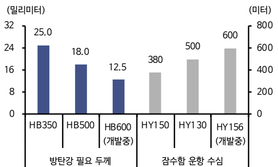
방위산업용 특화 강재
