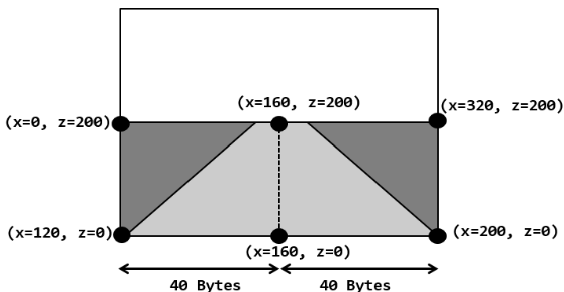
Fig. 101 coordenadas del mundo proyectadas
