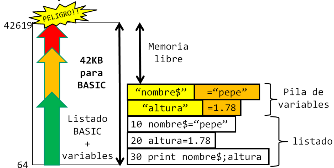
Fig. 8 Crecimiento del consumo de memoria de listado BASIC y variables
