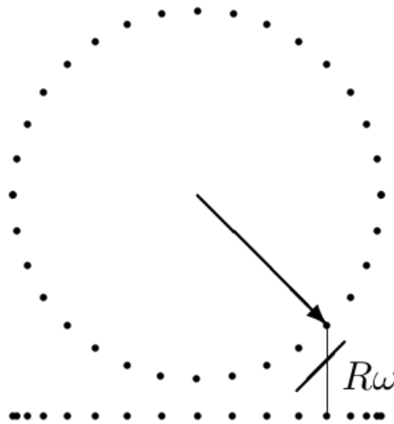
Figura 1.4: circunferencia de radio R recorrida con velocidad angular \omega en sentido horario; la proyecci3n sobre el eje x ejecuta movimiento arm3nico simple.
