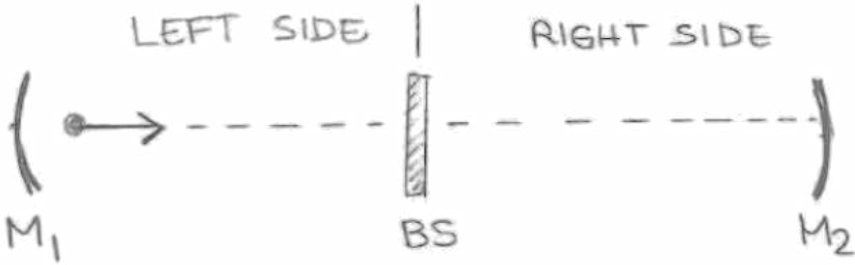
Figura: una cavidad con el divisor de haz BS entre dos espejos perfectamente reflectantes M_1 (izquierda) y M_2 (derecha); un fotón entra desde la izquierda hacia BS. Se indican el «lado izquierdo» y el «lado derecho» de la cavidad, separados por BS.
