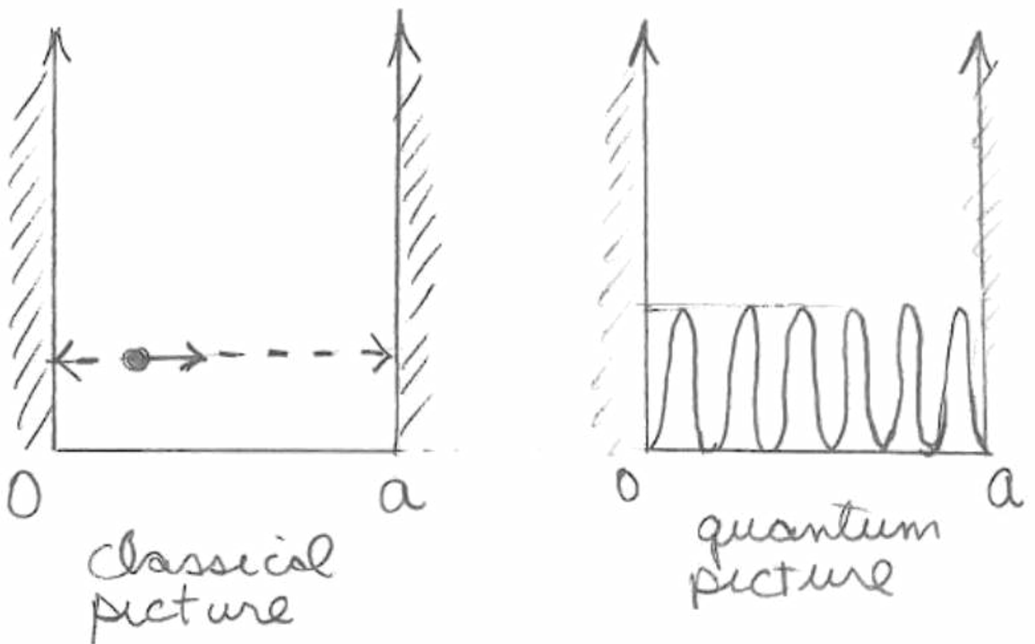
Figura 6: Partícula en una caja unidimensional. La partícula rebota con velocidad constante.
