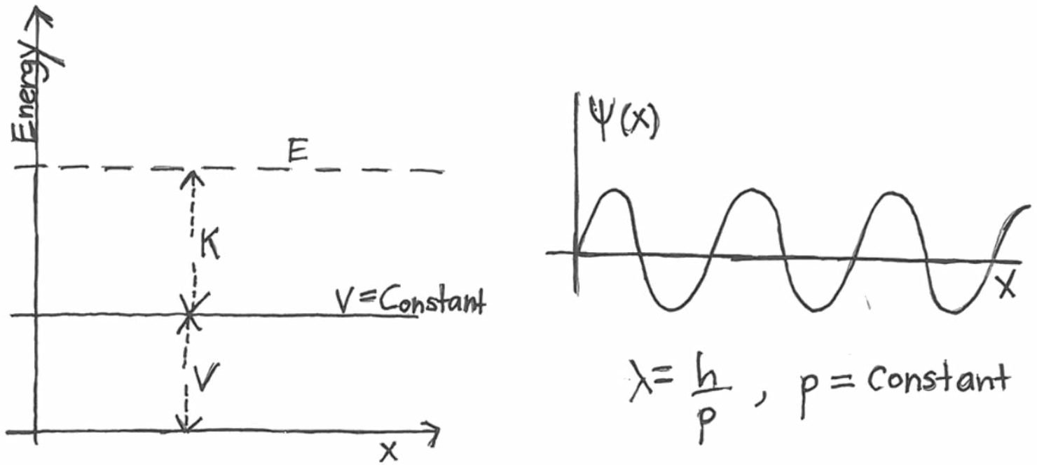
Figura 2: A la izquierda, un ejemplo de potencial constante, V = V_0 < E , donde K es la energía cinética y E = K + V_0 es la energía total. A la derecha, un esbozo de la función de onda para una partícula en este potencial. V constante \Rightarrow K constante, por tanto el momento también es constante.
