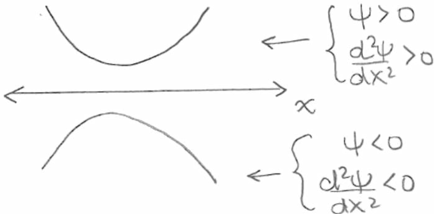
Figura 7: En la región clásicamente prohibida, o bien \psi > 0 , \psi'' > 0 , o bien \psi < 0 , \psi'' < 0 . En ambos casos la función de onda es convexa hacia el eje x .
