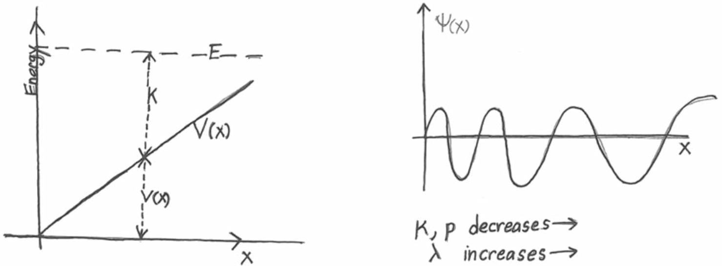
Figura 3: Un potencial que varía linealmente, V(x) = \alpha x . La energía E = K + V(x) es fija, y al aumentar x , K(x) disminuye, p(x) disminuye y \lambda(x) aumenta, resultando en una función de onda de longitud de onda creciente.
