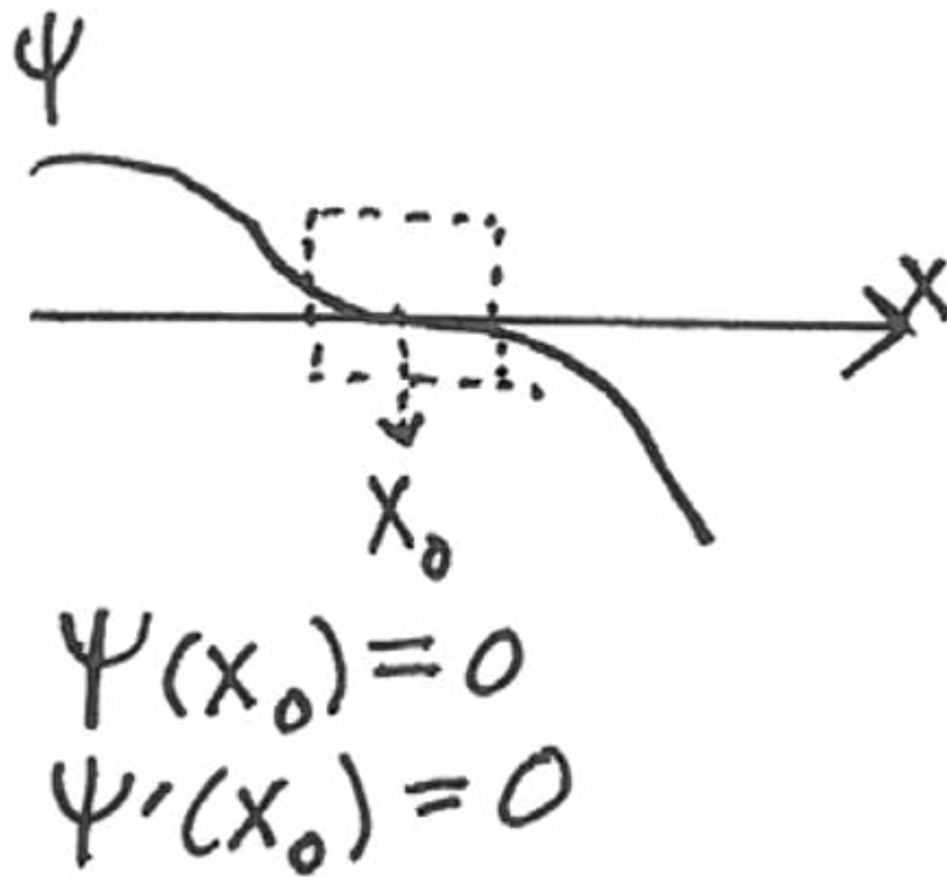
Figura 10: Es imposible que tanto \psi como \psi' se anulen en algún punto x_0 : la ecuación de Schrödinger obligaría entonces a que \psi(x) se anule idénticamente.
