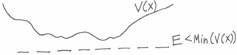
Figura 1: No existen soluciones con energía E menor que el mínimo del potencial V(x) .
