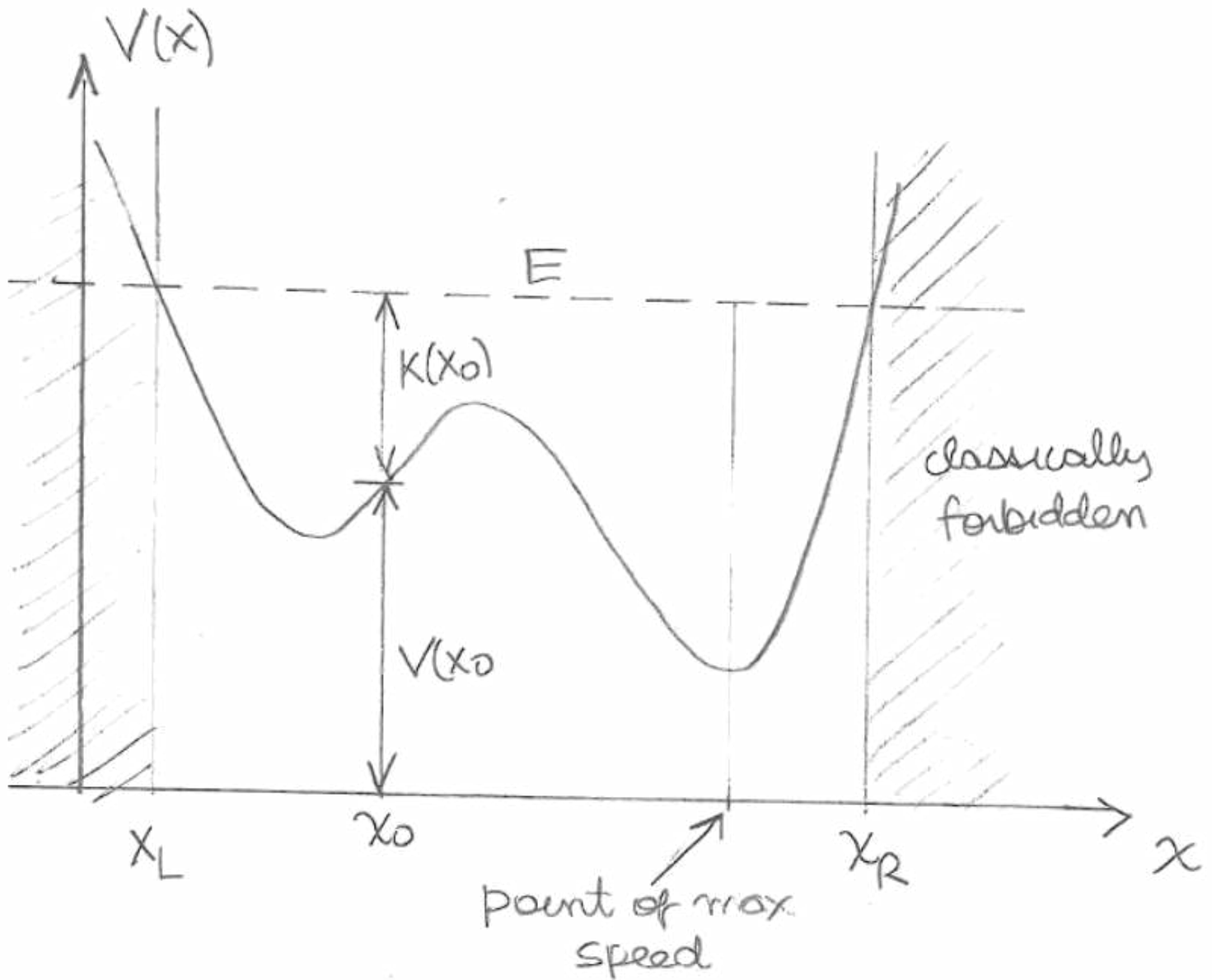
Figura 4: Un potencial arbitrario que muestra los puntos de retorno x_L y x_R . La región a la derecha de x_R y la región a la izquierda de x_L son regiones clásicamente prohibidas. En cualquier punto x \in [x_L, x_R] la suma de la energía potencial V(x) y la energía cinética K(x) es igual a la energía total E .
