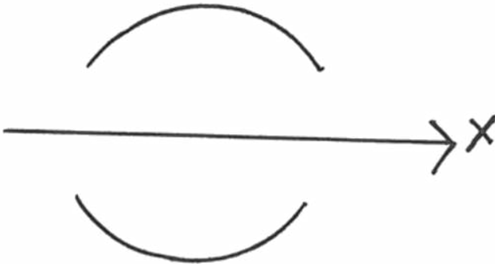
Figura 9: \psi > 0 , \psi'' < 0 , o \psi < 0 , \psi'' > 0 . La función de onda es cóncava hacia el eje x .
