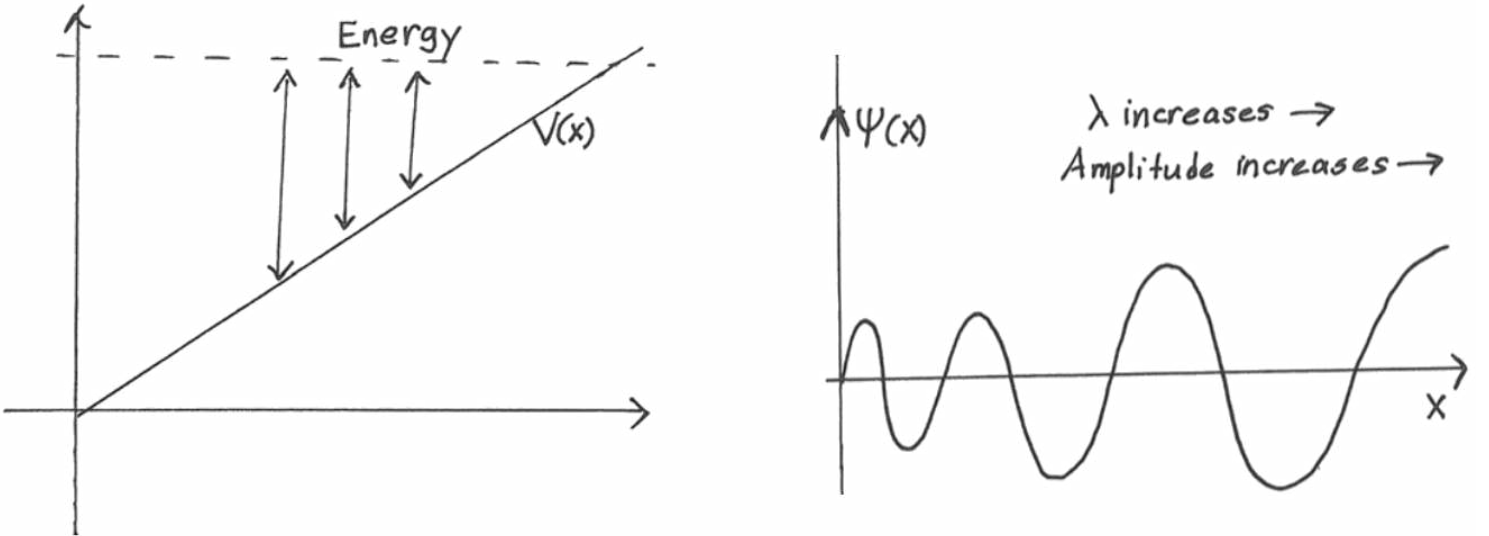
Figura 5: Un potencial V(x) y una energía cinética que disminuye al aumentar x . Entonces la longitud de onda de de Broglie aumenta con x . La ecuación 2.8 implica entonces que la amplitud de \psi(x) también aumenta con x .
