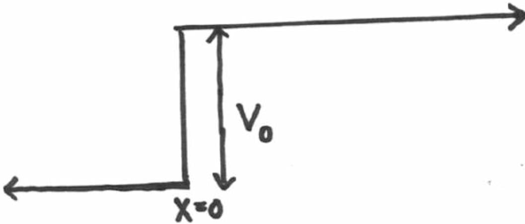
Figura 1: El potencial escalón.
