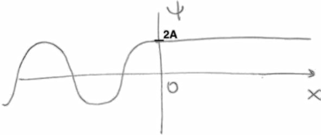
Figura 3: Estado propio de energía para E = V_0 .
