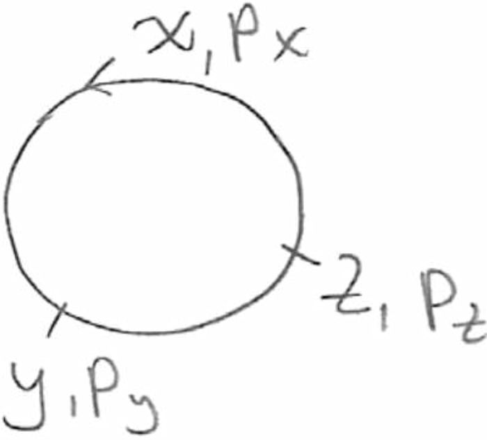
Figura 1: Las relaciones de conmutación del momento angular satisfacen la ciclicidad.
