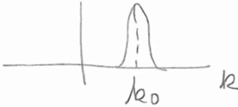
Figura 2: Se supone que la función \Phi(k) tiene un pico alrededor de k = k_0 .
