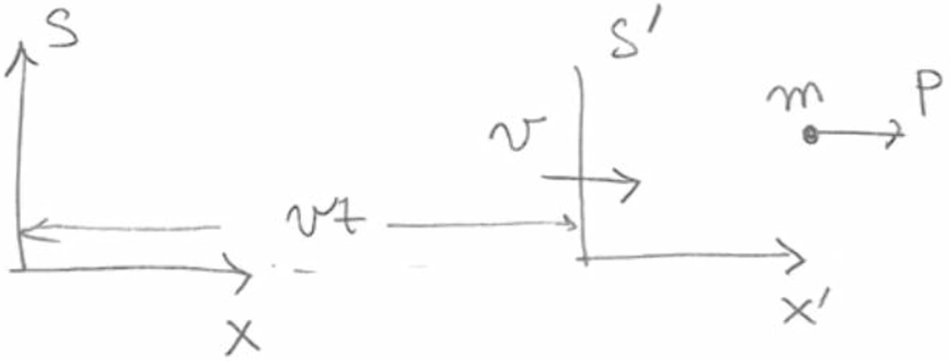
Figura 1: El referencial S' se mueve con velocidad v a lo largo de la dirección x del referencial S . Una partícula de masa m se mueve con velocidad \tilde{v} , y por lo tanto con momento p = m\tilde{v} , en el referencial S .
