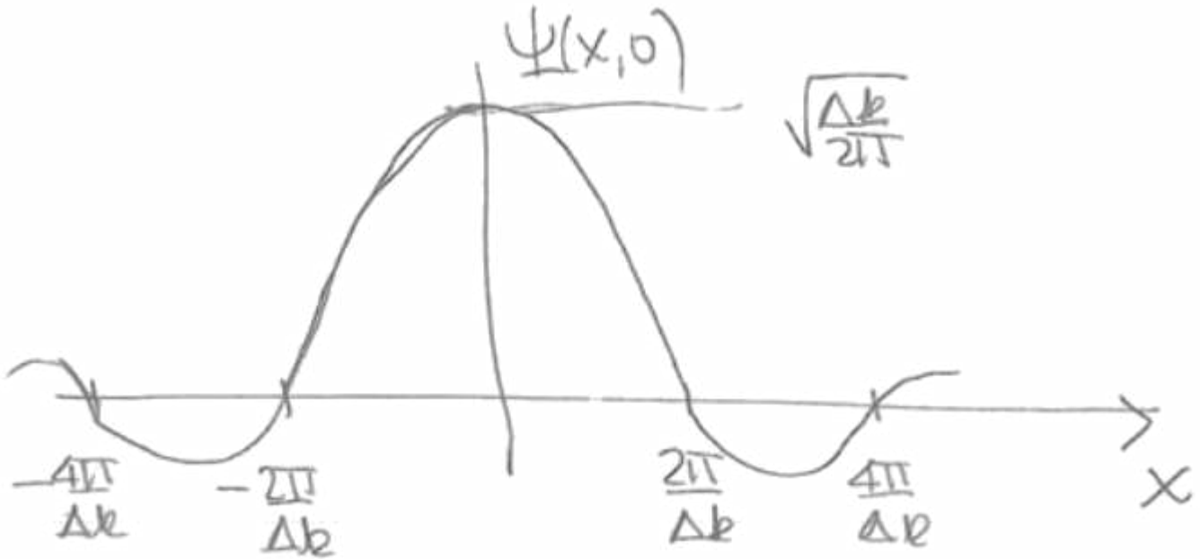
Figura 5: La \Psi(x, 0) correspondiente a la \Phi(k) .
