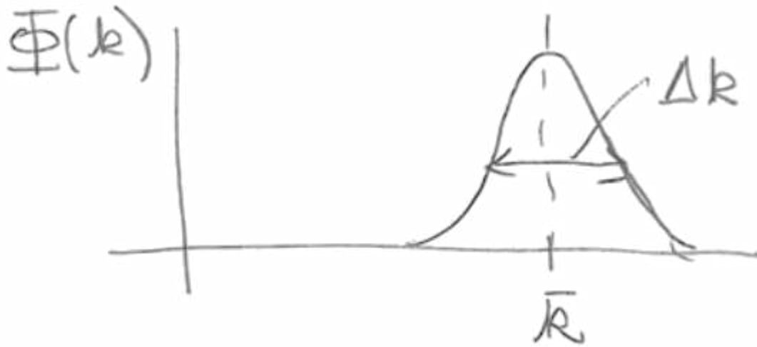
Figura 1: Una \Phi(k) centrada en k = k_0 y con anchura \Delta k .
