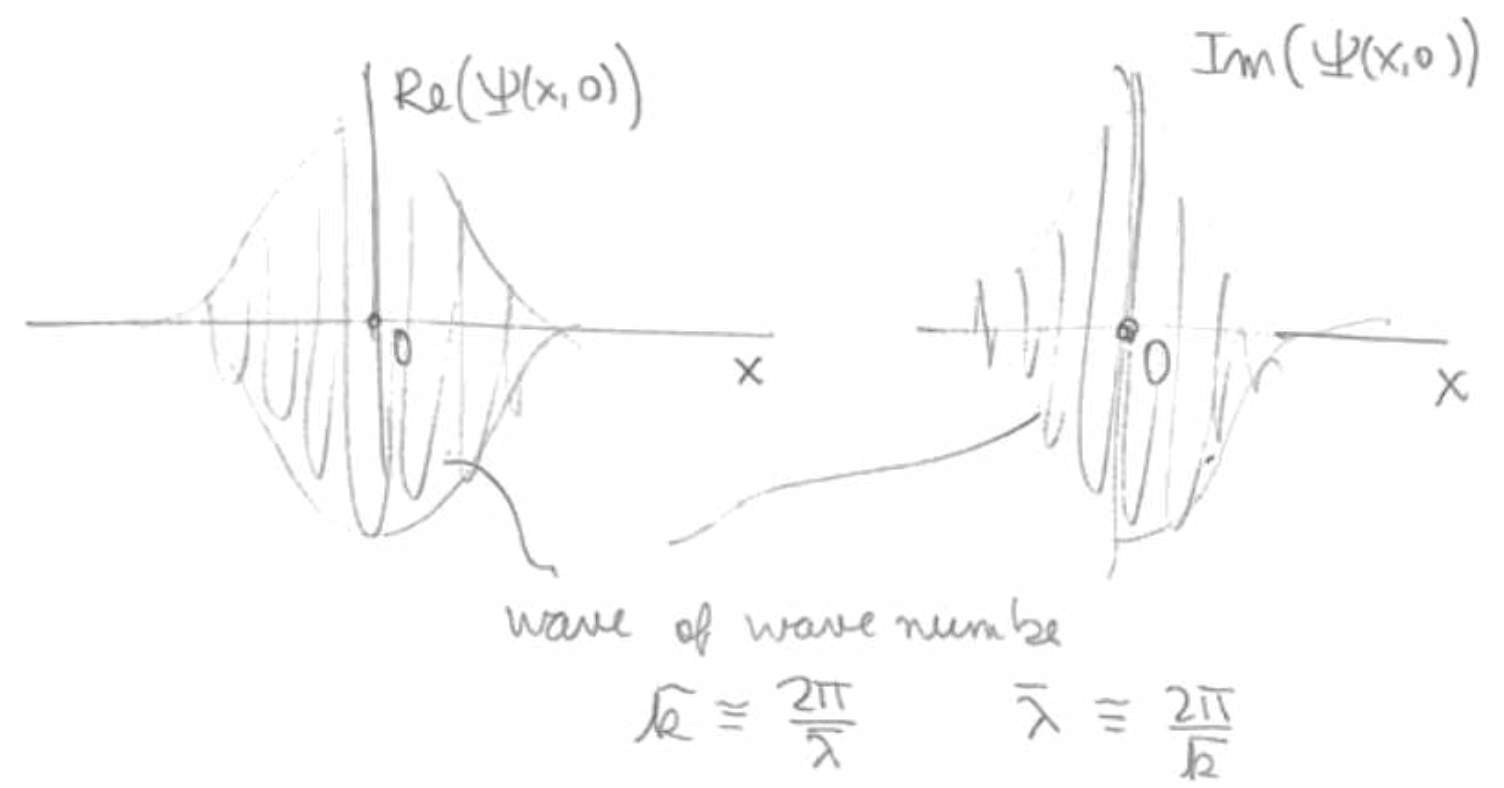
Figura 3: Las partes real e imaginaria de \Psi(x, 0) .
