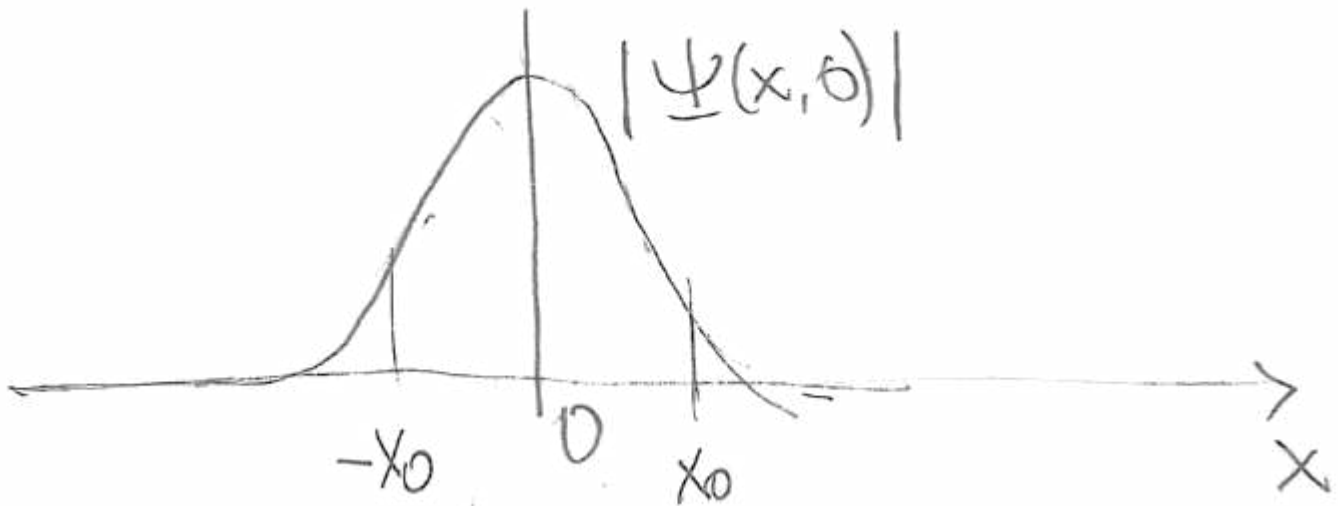
Figura 2: La \Psi(x, 0) correspondiente a la \Phi(k) mostrada en la Fig. 1, centrada en x = 0 con anchura \Delta x .
