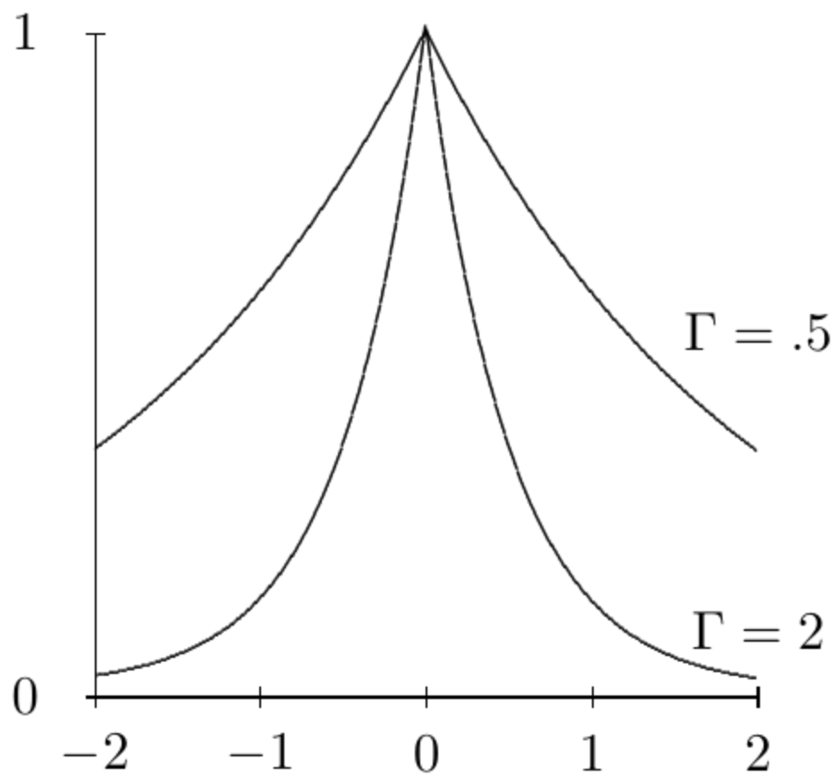
Figura 10.4: f(t) = e^{-\Gamma|t|} para \Gamma = 0.5 y \Gamma = 2 .
