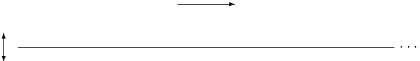
Figura 10.1: una cuerda semiinfinita.
