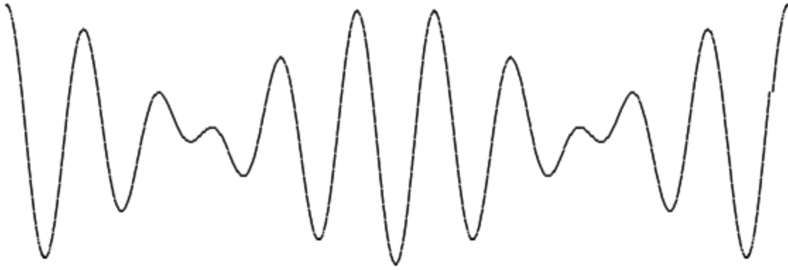
Figura 10.3: la función (10.21) para t = 0 y k_0/k_s = 10 .
